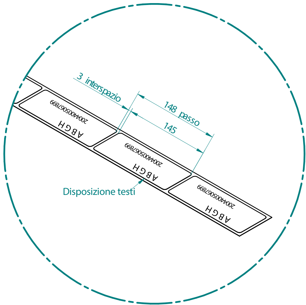
DETTAGLIO A
